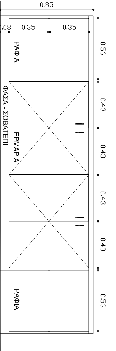
ΟΨΗ - ΚΛ.1:20
