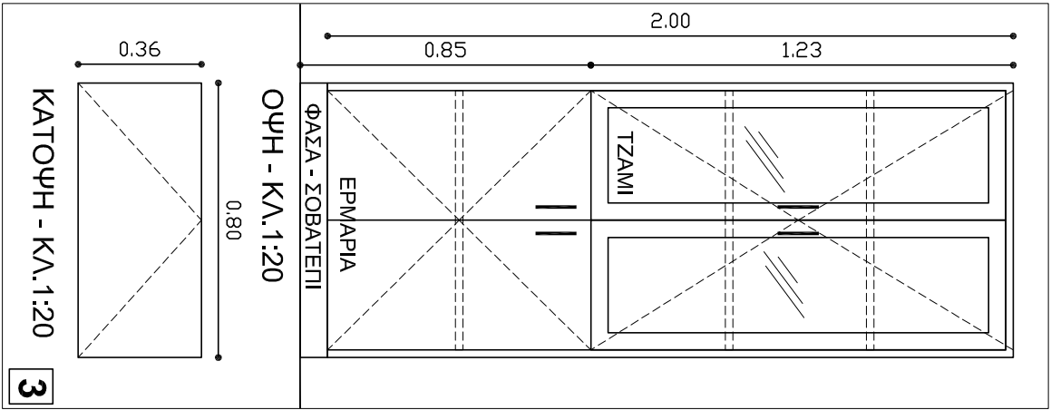
ΚΑΤΟΨΗ - ΚΛ.1:20
