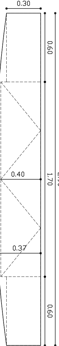
ΟΨΗ - ΚΛ.1:20
