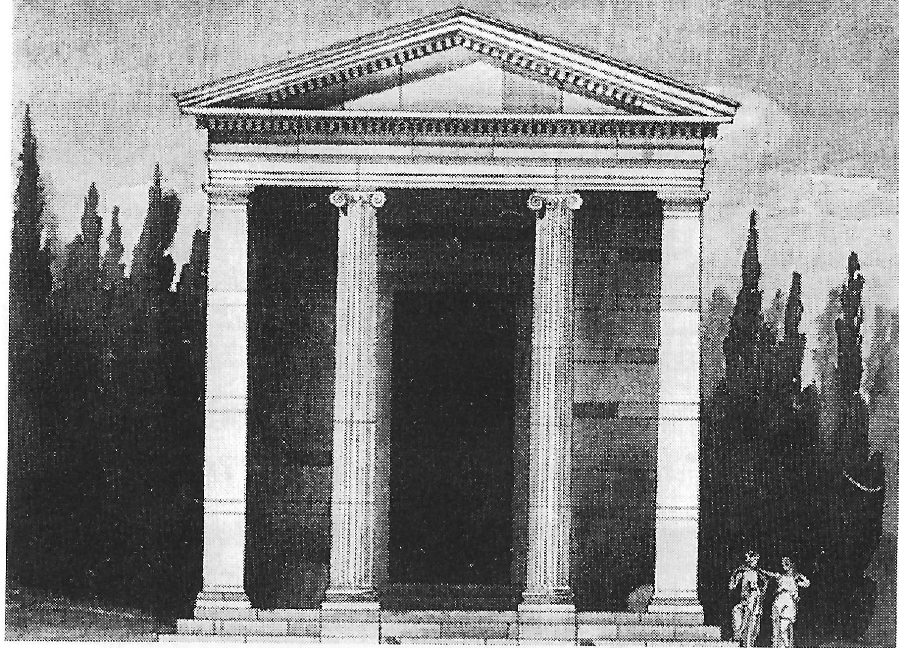
334. Κως, Ασκληπιείο. Ιωνικός ναός του Ασκληπιού (1:200).
