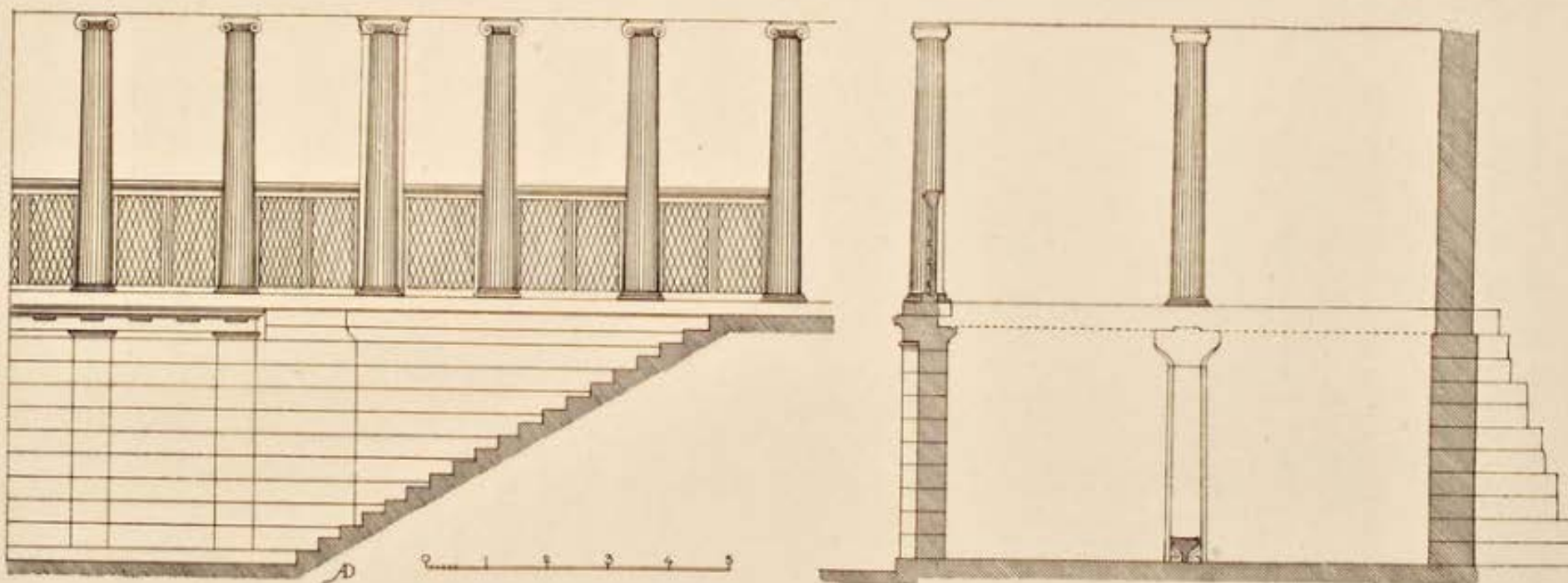
DEUXIÈME PORTIQUE ET SALLE BASSE. (Coupe et élévation restaurées.)
