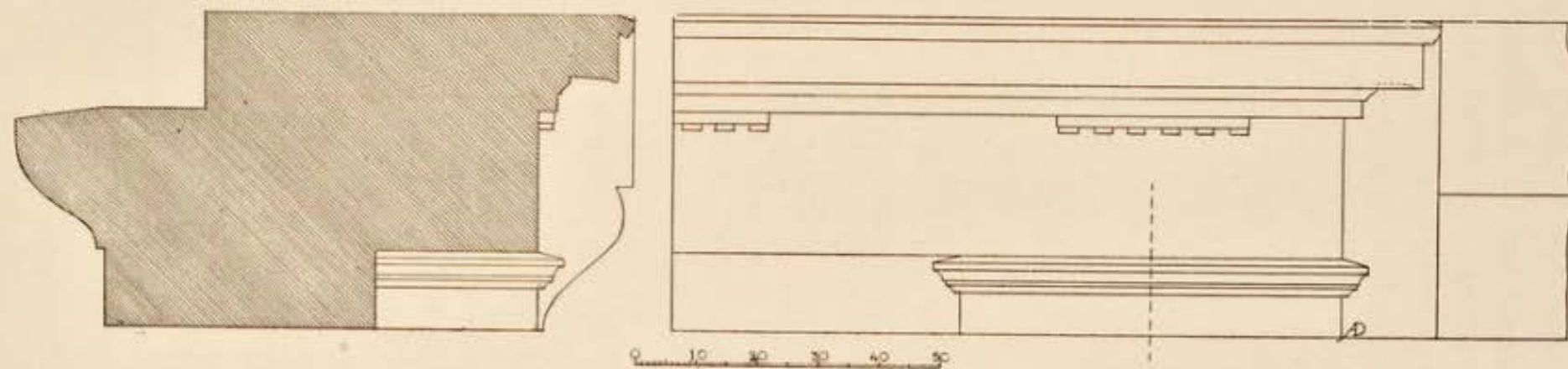
FAÇADE DE LA SALLE BASSE. (Détail de l'entablement.)
